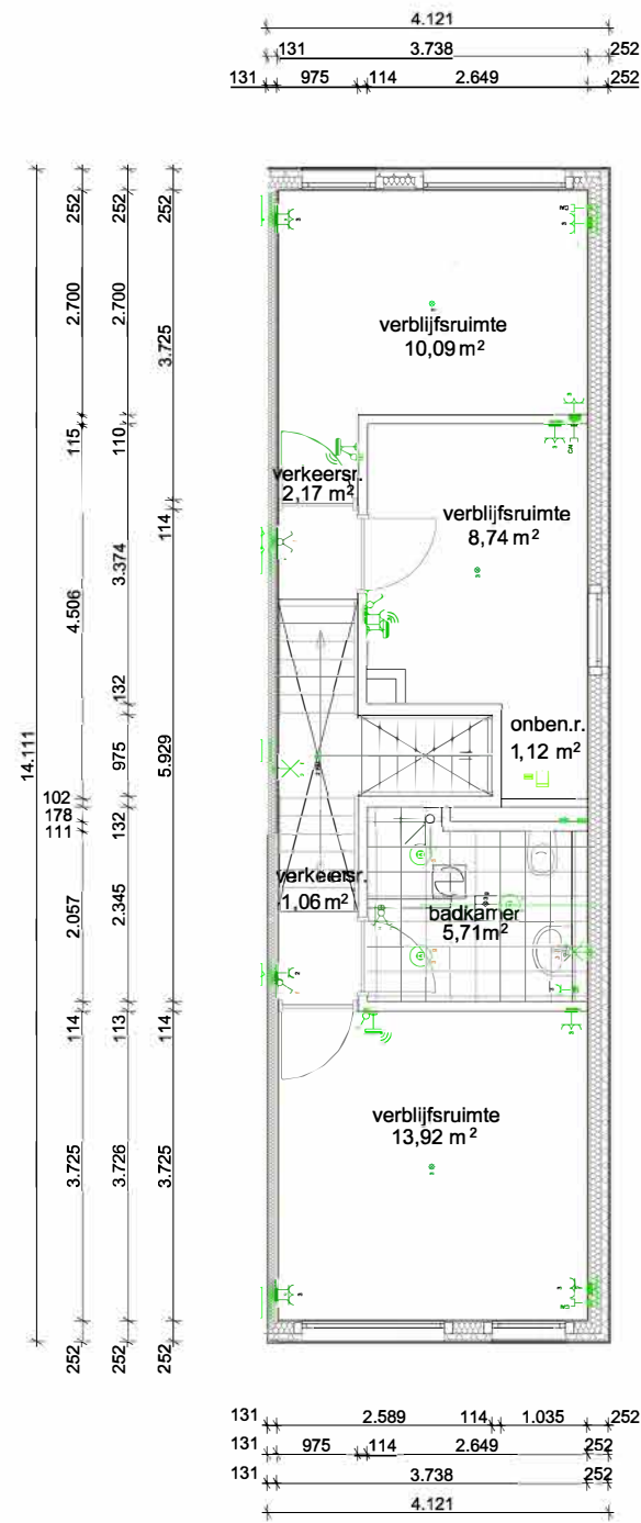
Verdieping
