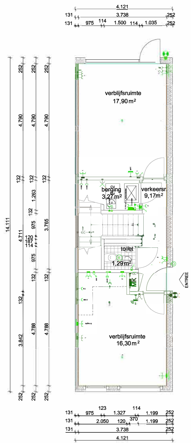
Begane grond
